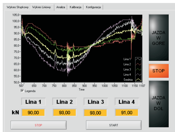
Aplikacja serwisowa kontroli stanu pracy urządzenia
